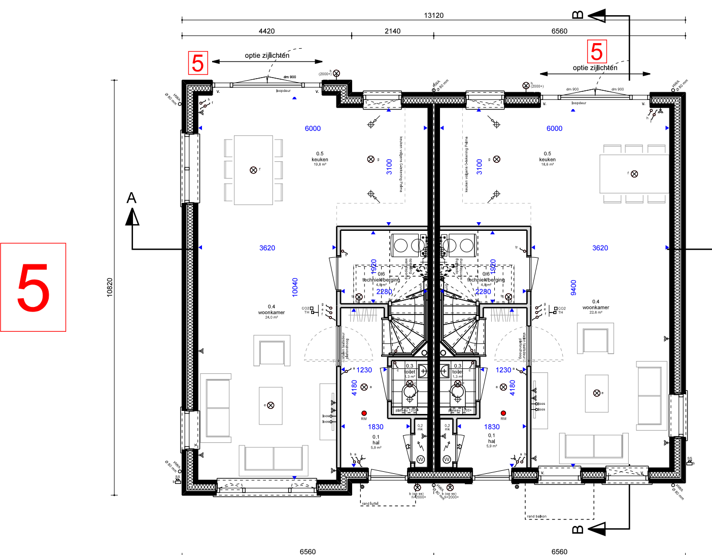
BEGANE GROND (optie 5)
