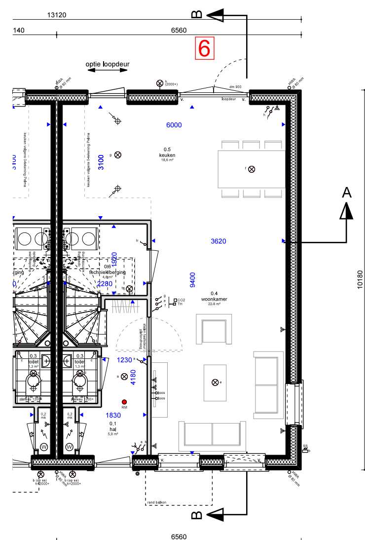
BEGANE GROND (optie 6)
