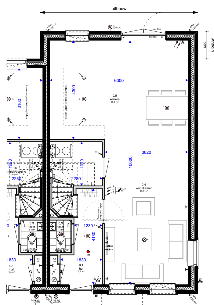
BEGANEGROND (optie 4)
