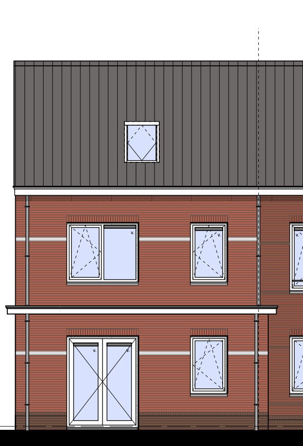
ACHTERGEVEL
