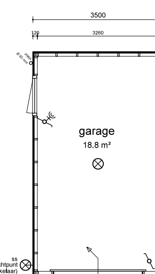
PLATTEGROND nummer 26
