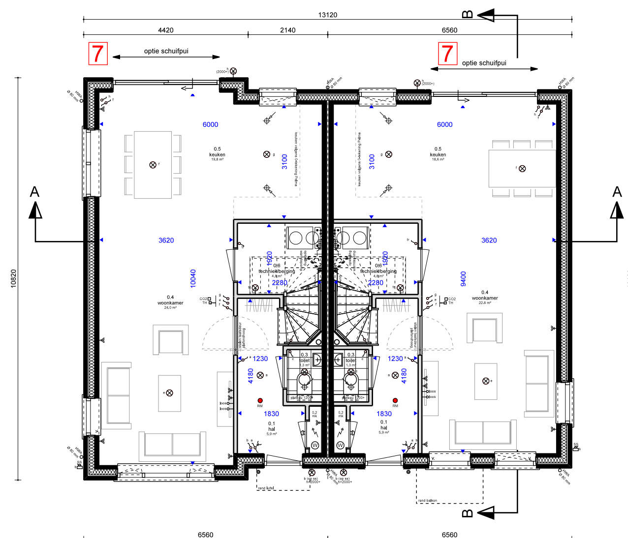
BEGANE GROND (optie 7)
