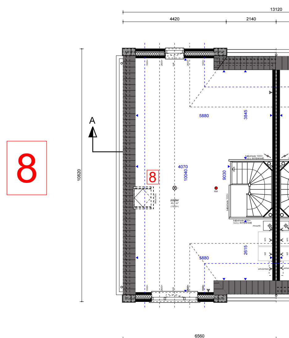
ZOLDER (optie 8)
