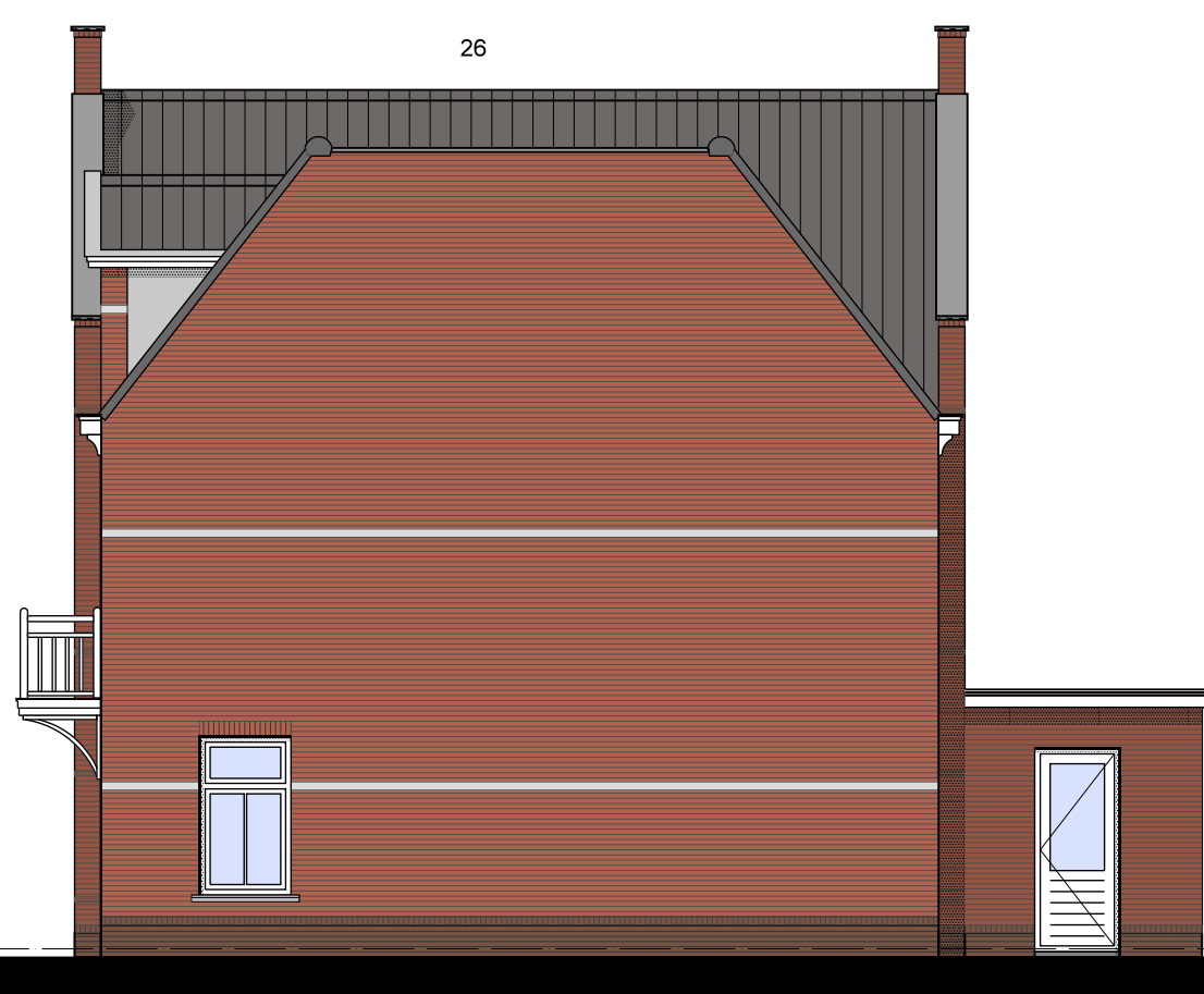
RECHTERGEVEL
