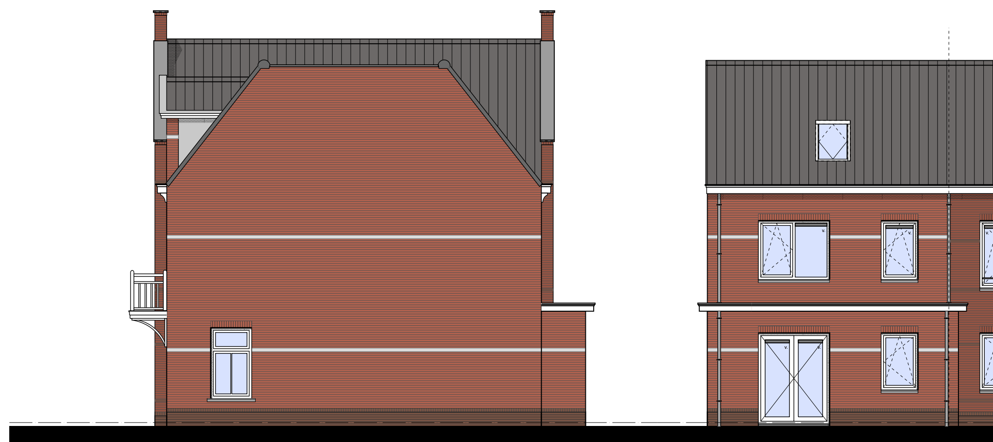
RECHTERGEVEL (optie 4)
