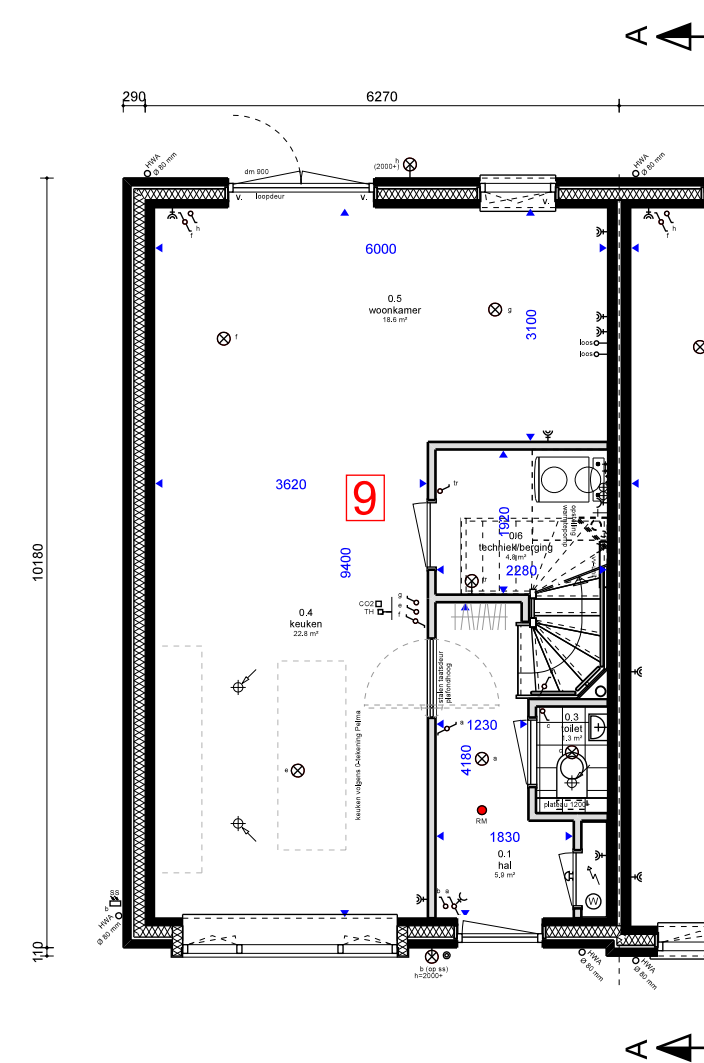
BEGANE GROND (optie 9) nr. 27 t/m 30 en 33 t/m 38
