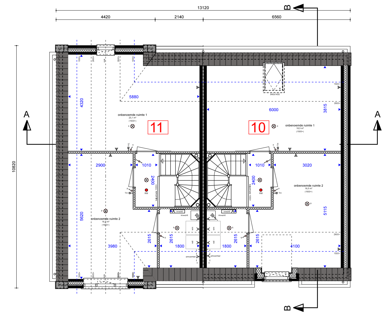
ZOLDER (optie 10, 11 en 12)
