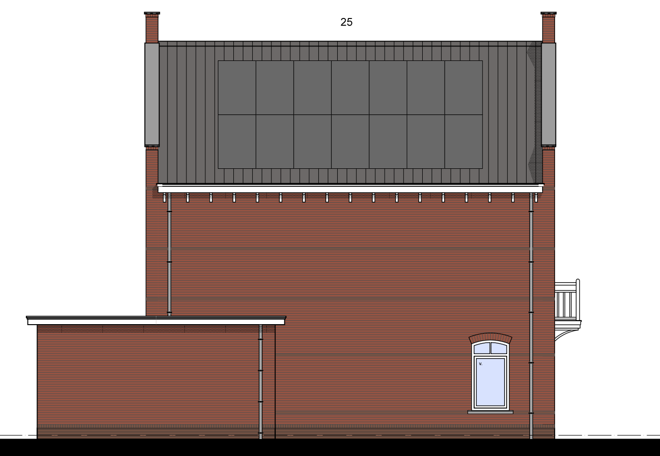
LINKERGEVEL
