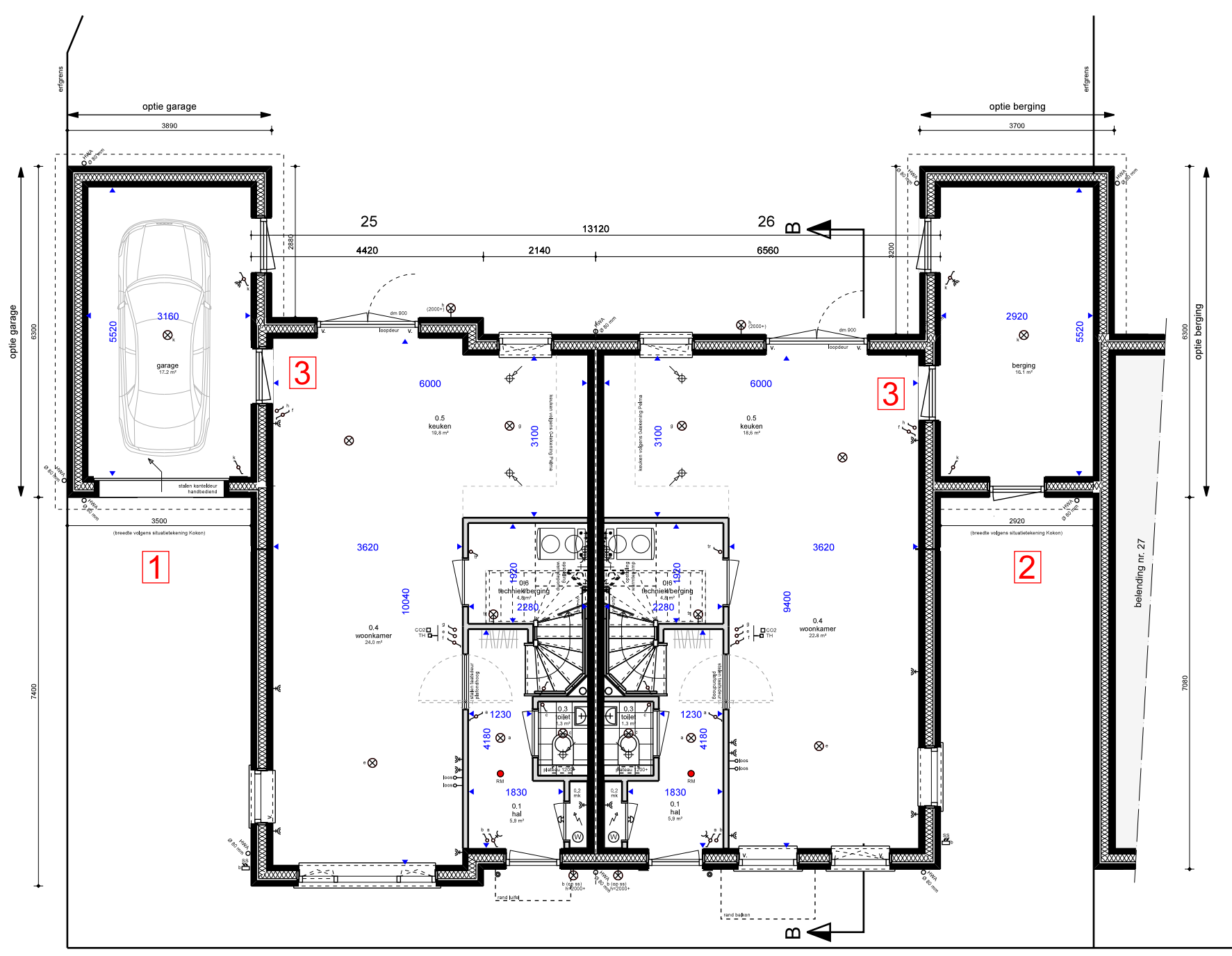
1 2 3 BEGANEGROND (optie 1, 2 en 3)
